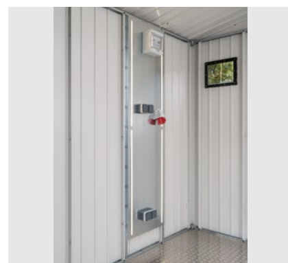
Elektrisch paneel incl. stopcontacten, licht en optionele krachtstroomaansluiting
