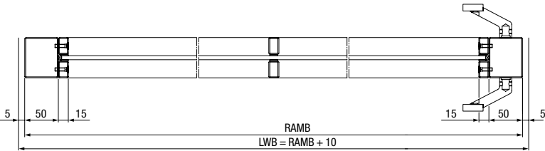
Horizontale doorsnede pivotdeur in standaarduitvoering, symmetrische verdeling van de dwarsstijlen
