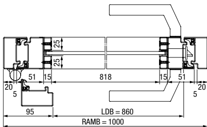
Horizontale doorsnede 1-vleugelige draaivleugeldeur
