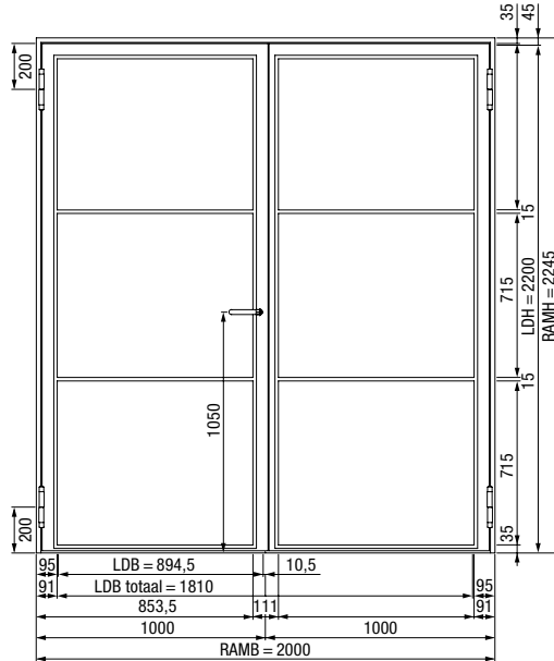
2-vleugelige draaivleugeldeur
