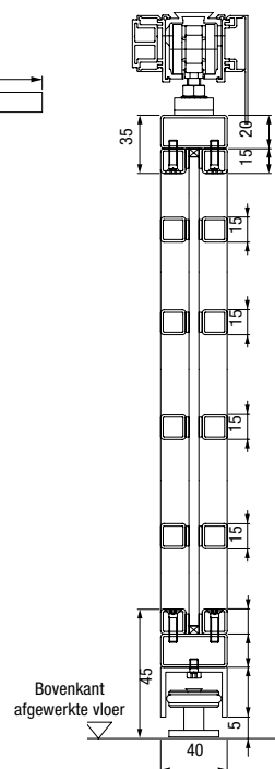
Verticale doorsnede
