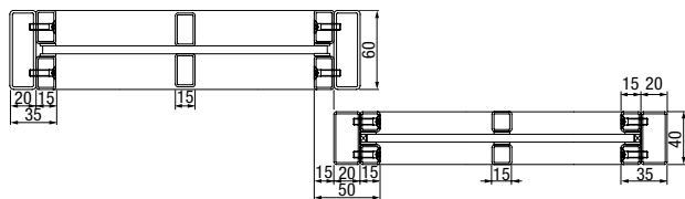
Horizontale doorsnede
