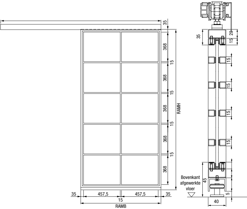
1-vleugelige schuifdeur
