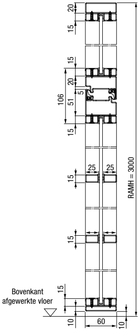
Verticale doorsnede
