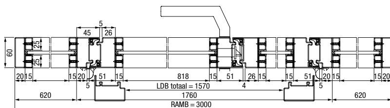
Horizontale doorsnede
