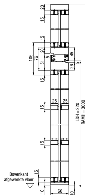
Verticale doorsnede
