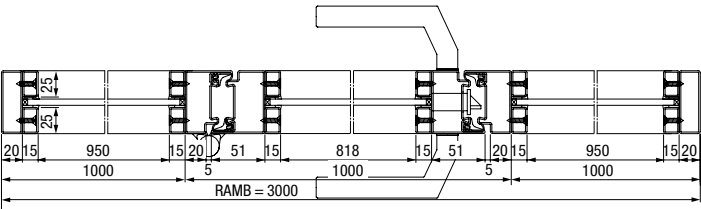
Horizontale doorsnede
