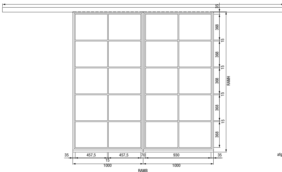
2-vleugelige schuifdeur
