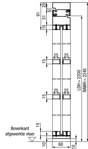
Verticale doorsnede
