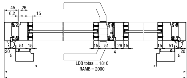
Horizontale doorsnede 2-vleugelige draaivleugeldeur
