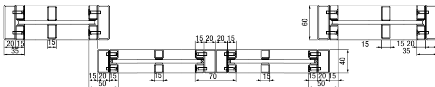
Horizontale doorsnede
