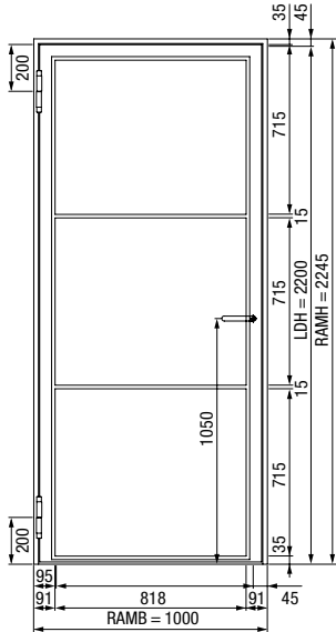
1-vleugelige draaivleugeldeur
