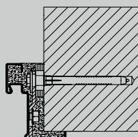
Hoekkozijn met verdoken plugmontage
