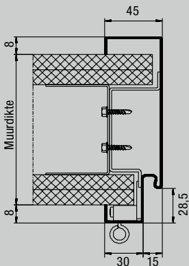
Profiel 21120
