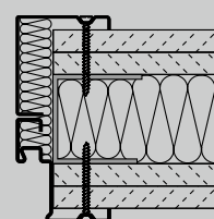
Hoek- en tegenkozijn Schroefmontage
