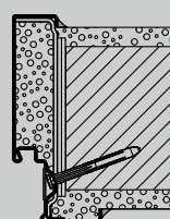
Muromvattend kozijn Diagonale bevestiging tot muurdikte 175
