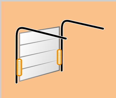
Ferrure Z : ferrure à ressorts de traction avec technique à ressorts de traction
